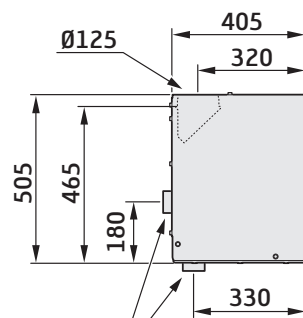
Røgrørstilslutning - top
